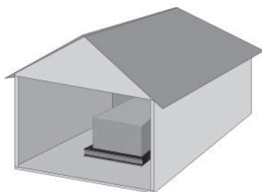
Armazenagem de placas cimentícias. O empilhamento máximo permitido é de 4 paletes.
